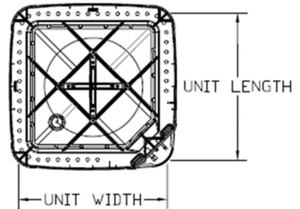
3 BOTTOM VIEW 9 N.T.S.
