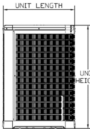
6 SIDE VIEW 9 N.T.S.
