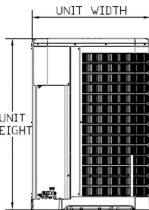
5 SIDE VIEW 9 N.T.S.
